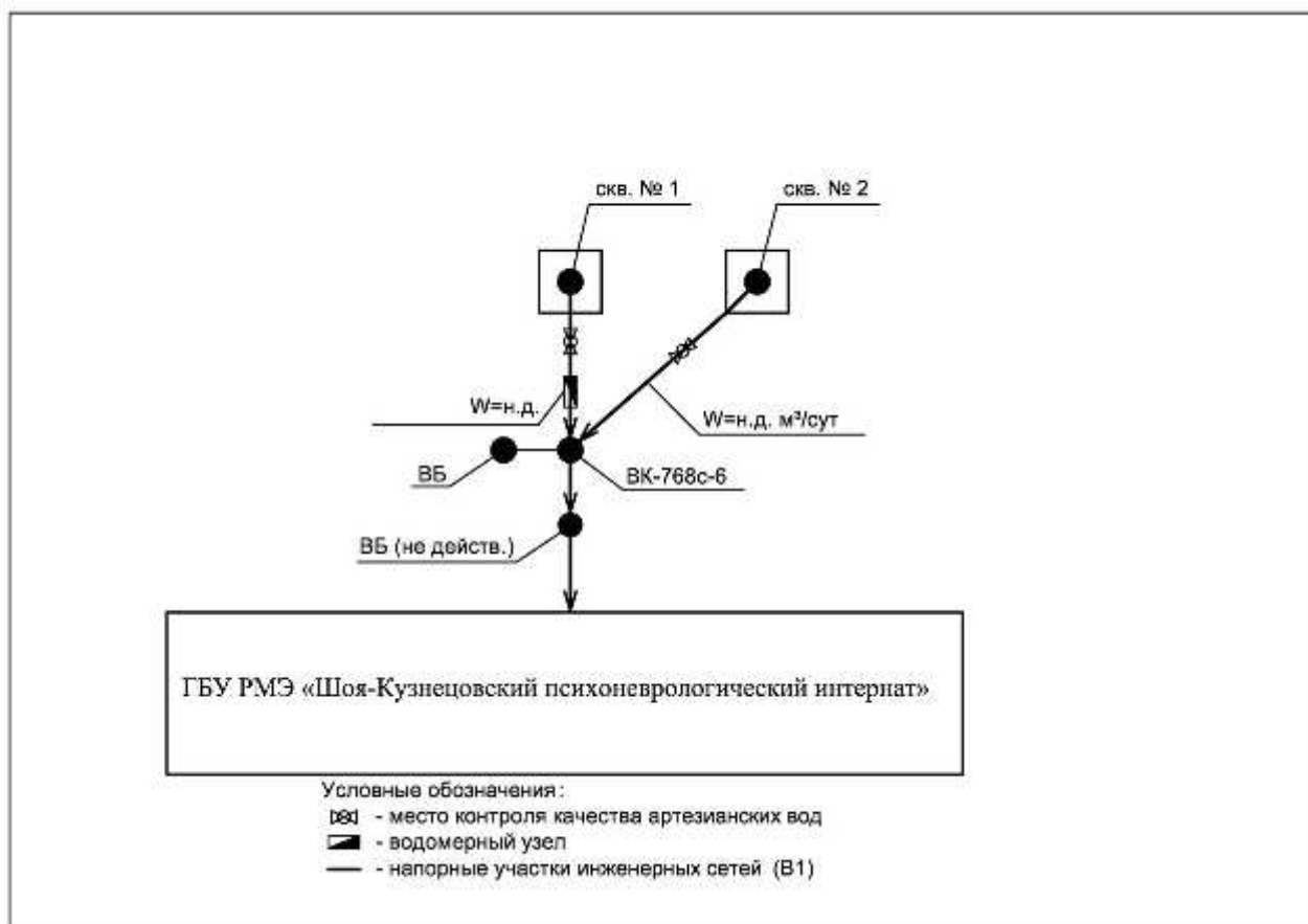
Рисунок 1.1.11. Принципиальная схема централизованной системы водоснабжения ГБУ РМЭ «Шоя-Кузнецовский ПНИ»
