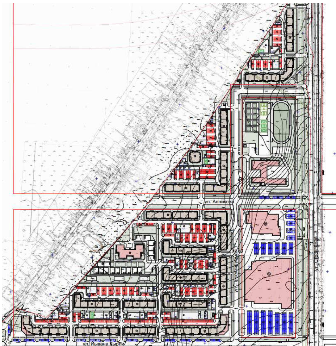
Рисунок 4.17. Схема микрорайона, ограниченного ул. Строителей, ул. Ийвана Кырлы и мкр. Мышино.
