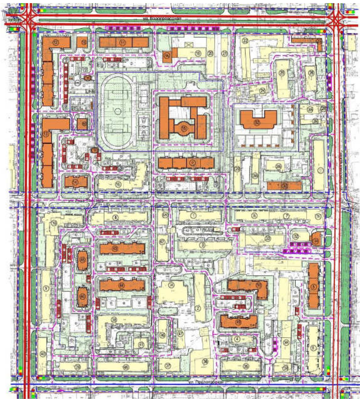
Рисунок 4.10 Схема микрорайона «Оршанский».
