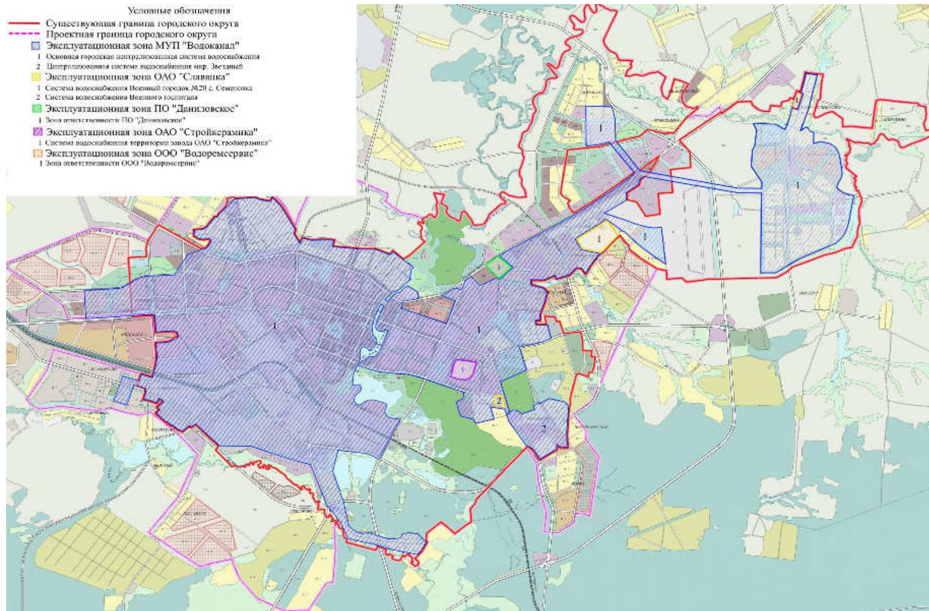
Рисунок 4.8.1. Границы планируемых зон размещения объектов централизованных систем водоснабжения
