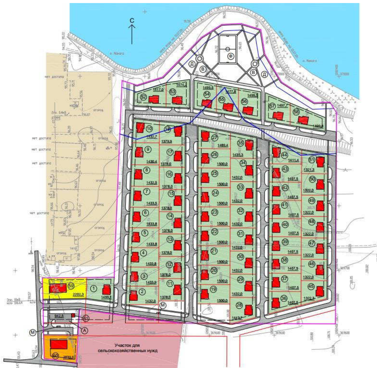
Рисунок 4.21 Схема участка под размещение жилых домов в районе деревни Апшакбеляк городского округа Йошкар-Ола.
